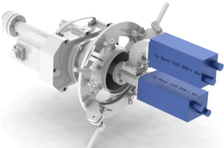
1.2.1.8 - Внешний вид ОУ Ку-диапазона № 6
