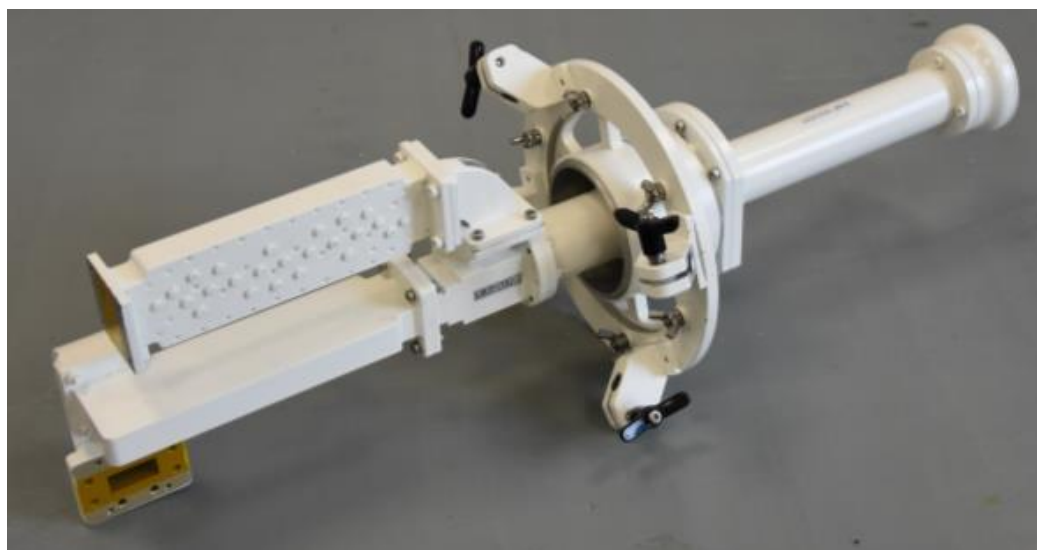
1.2.1.7 - Внешний вид ОУ X-диапазона № 5
