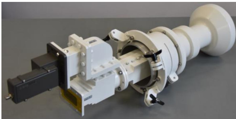
1.2.1.3 - Внешний вид ОУ С-диапазона № 2
