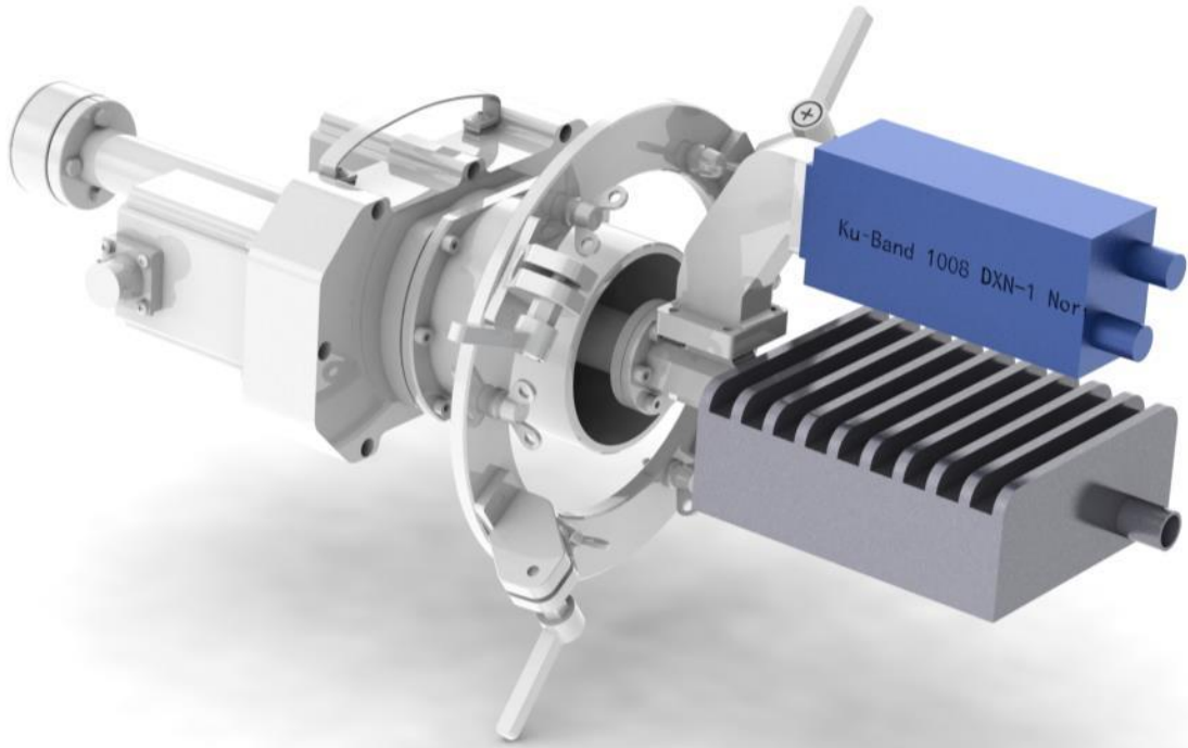
1.2.1.9 - Внешний вид ОУ Ку-диапазона № 7
