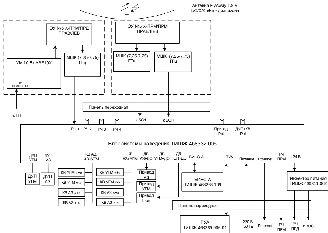
Рисунок 1.1.4.3 - Функциональная схема АП 1,8 м в комплектации Х-диапазона
