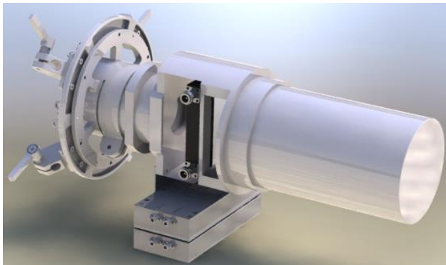
1.2.1.1 - Внешний вид ОУ L-диапазона
