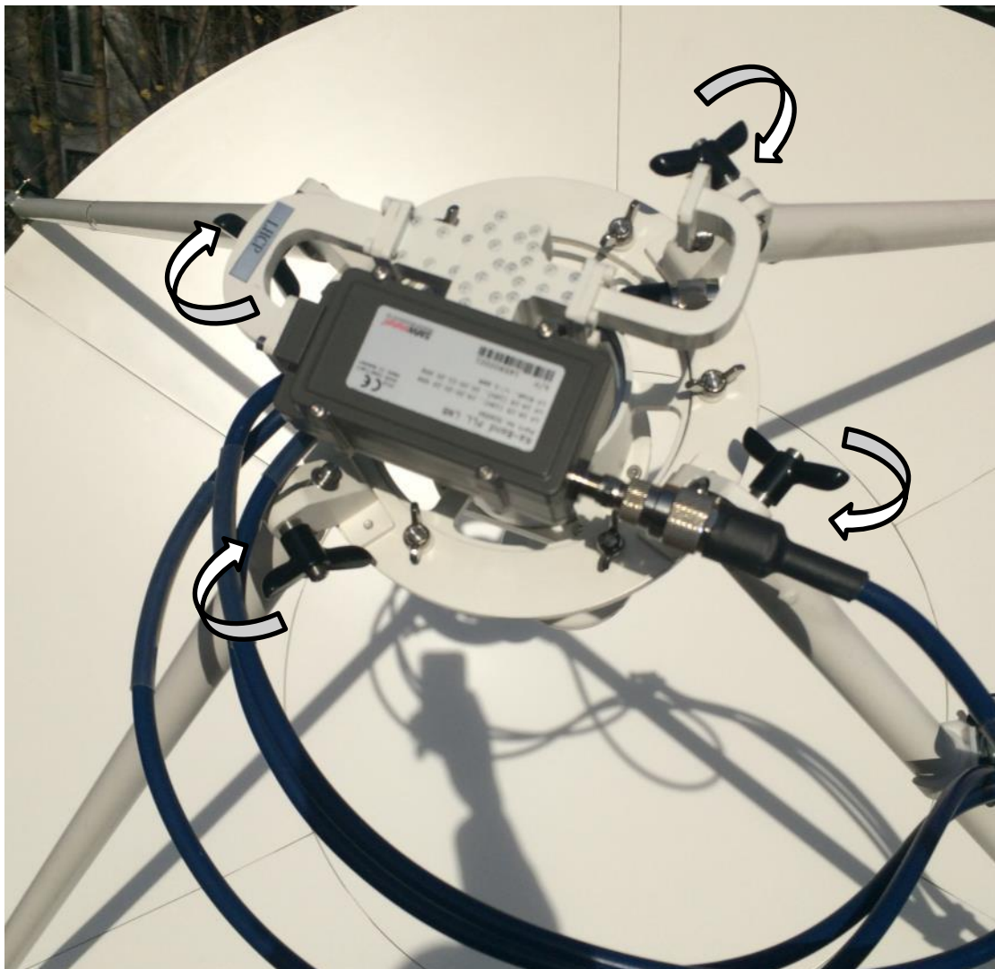
Рисунок 2.2.1.8.1 – Установка ОУ
