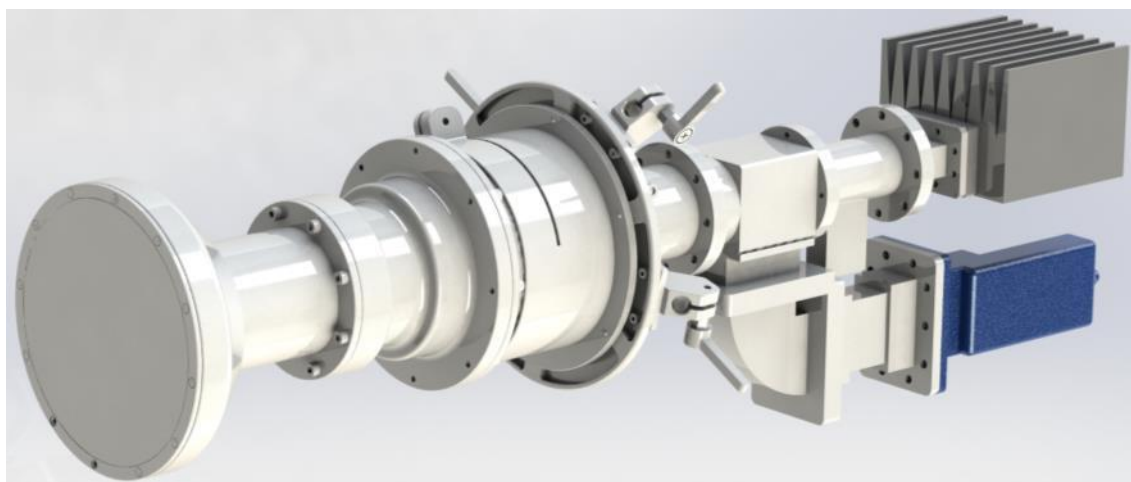
1.2.1.4 - Внешний вид ОУ С-диапазона № 3
