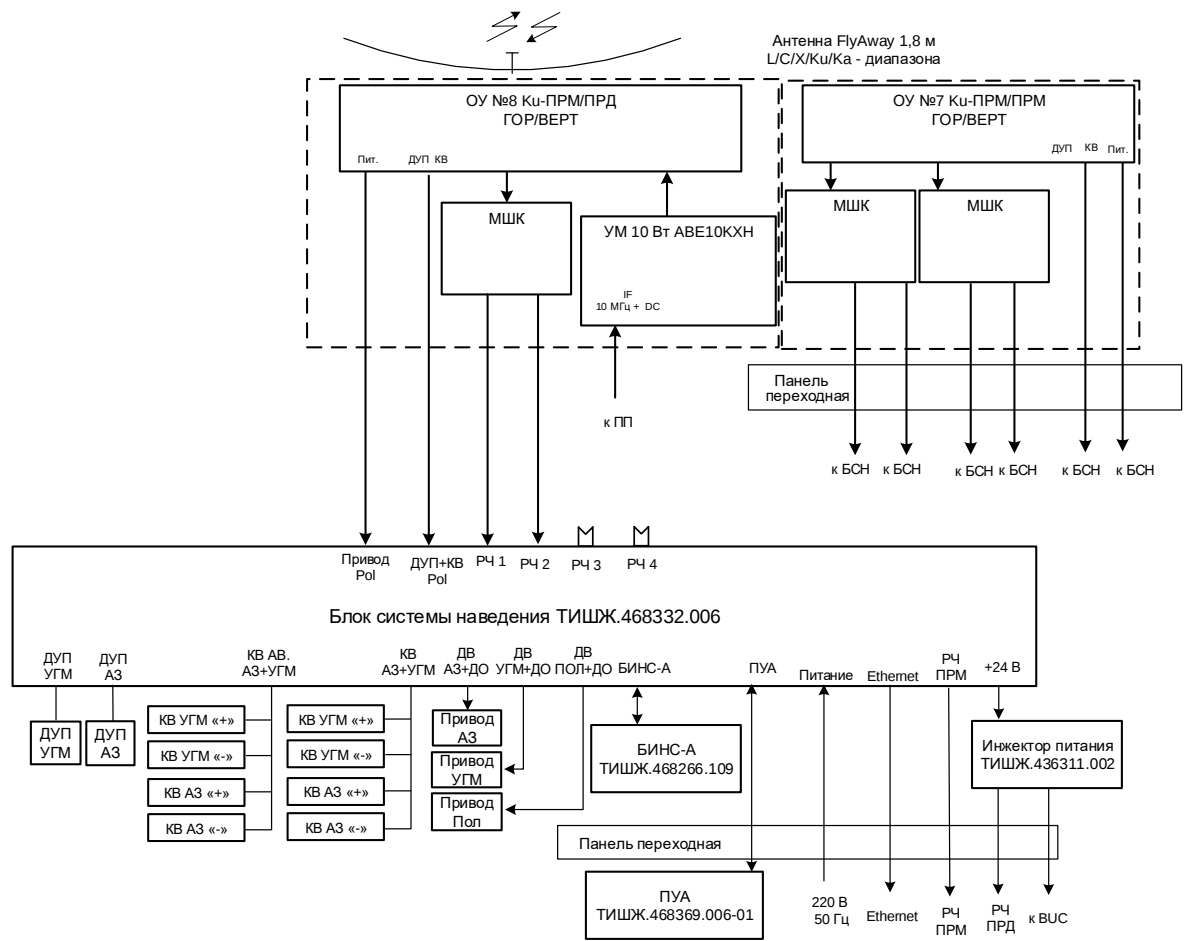
Рисунок 1.1.4.1 - Функциональная схема АП 1,8 м в комплектации Ku-диапазона
