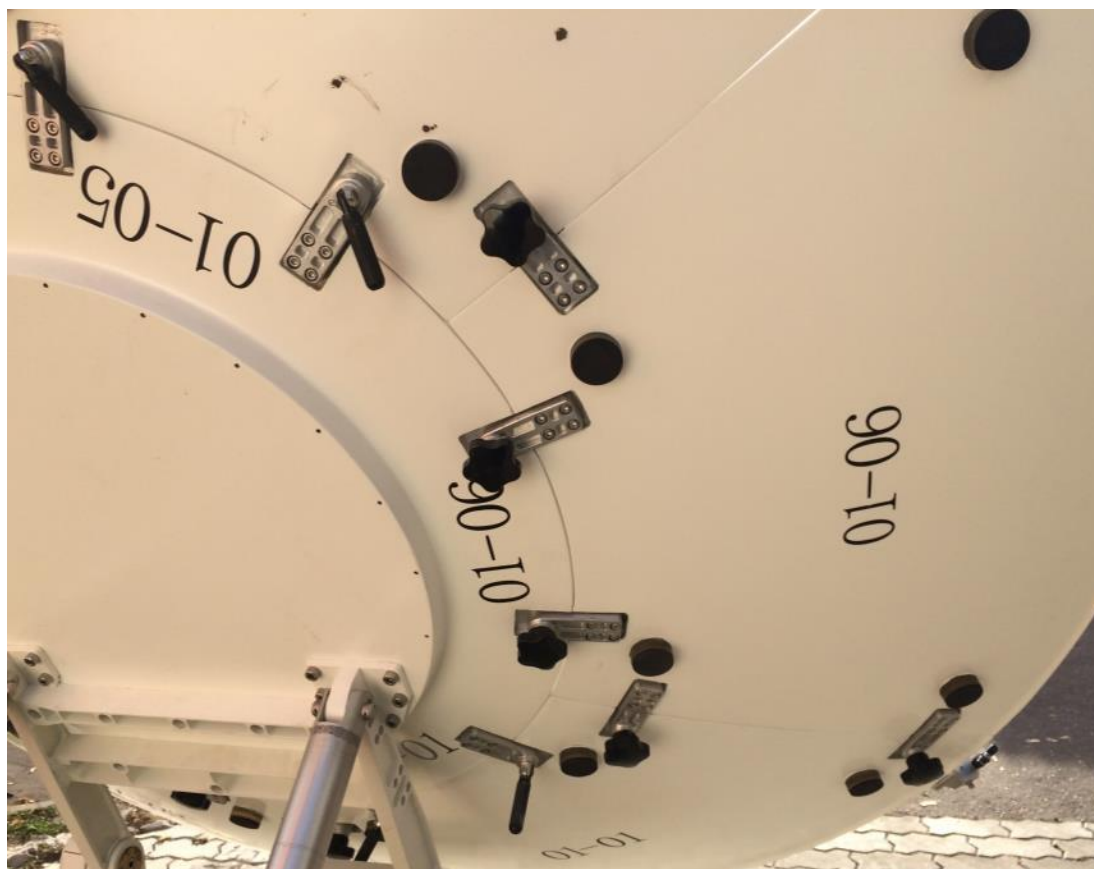
Рисунок 2.2.1.5.1 – Сборка антенны 1,8 м
