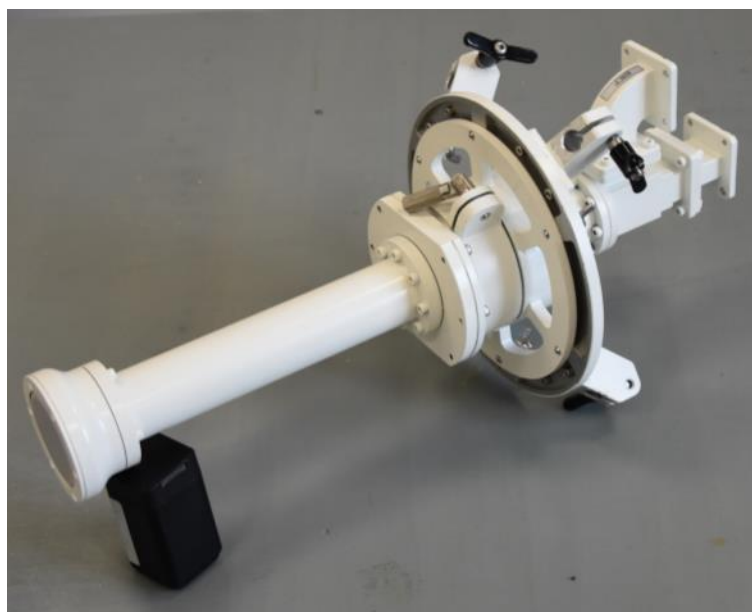
1.2.1.6 - Внешний вид ОУ Х-диапазона № 4
