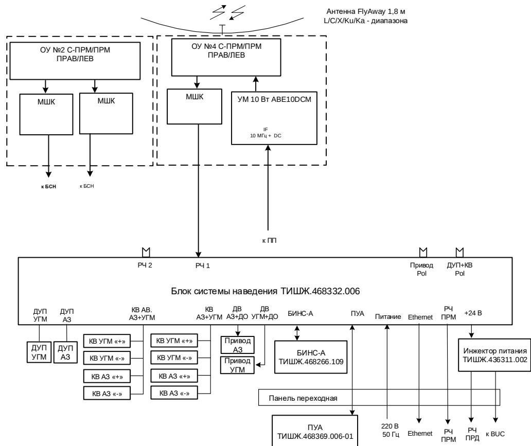
Рисунок 1.1.4.2 - Функциональная схема АП 1,8 м в комплектации С-диапазона
