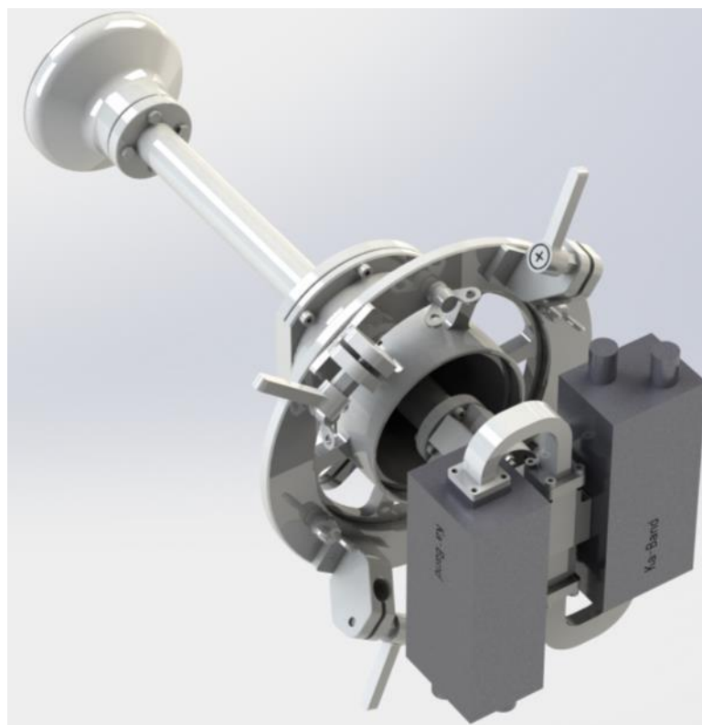
1.2.1.10 - Внешний вид ОУ Ка-диапазона № 8
