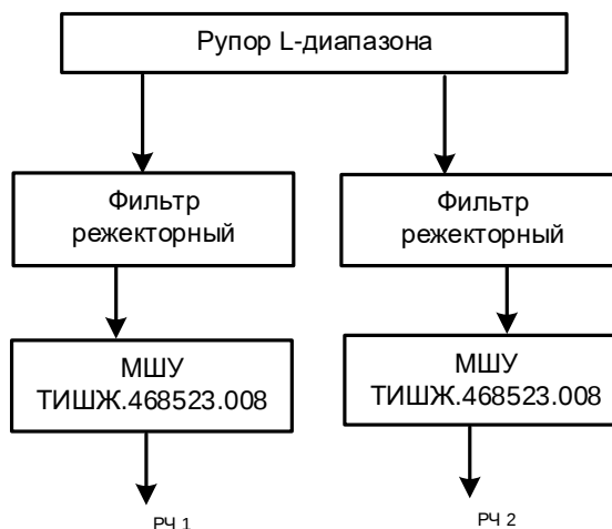
1.2.1.2 – Функциональная схема ОУ L-диапазона
